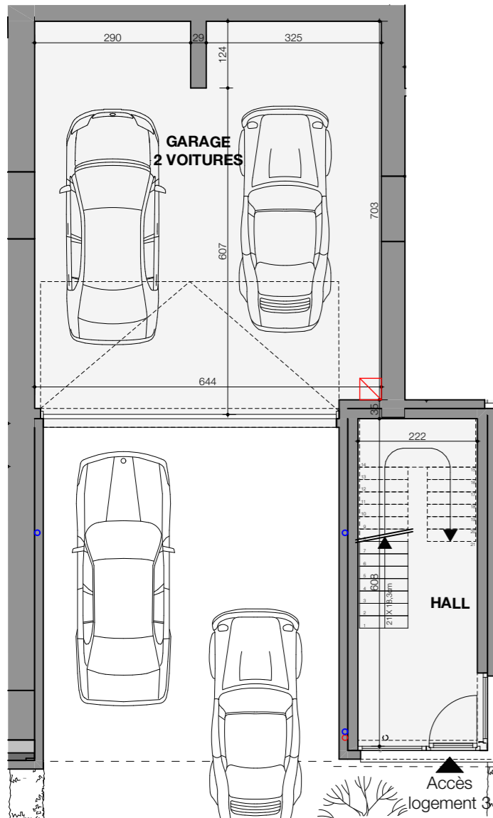
VUE EN PLAN SOUS-SOL
