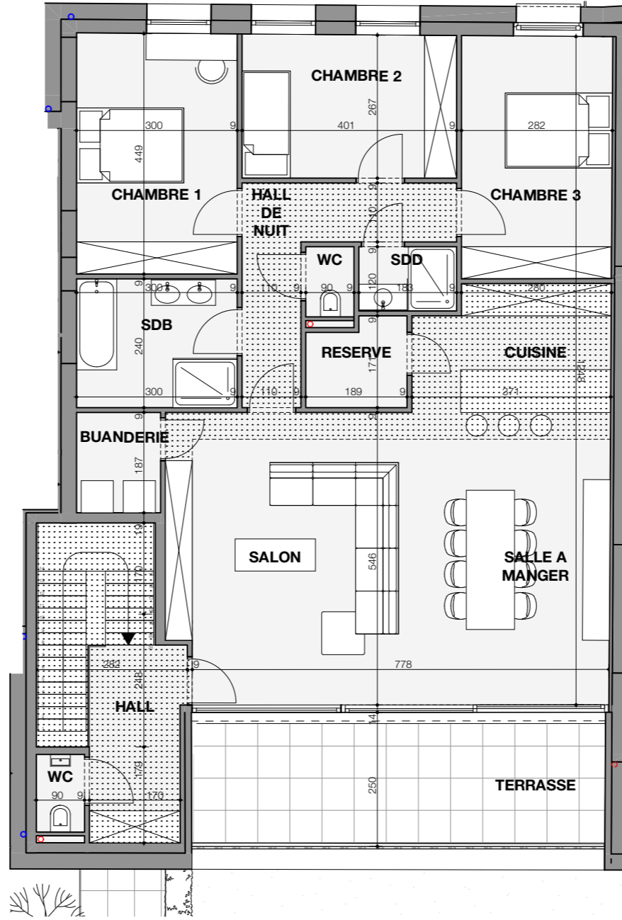
VUE EN PLAN REZ-DE-CHAUSSEE
