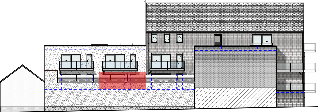
Façade jardin
