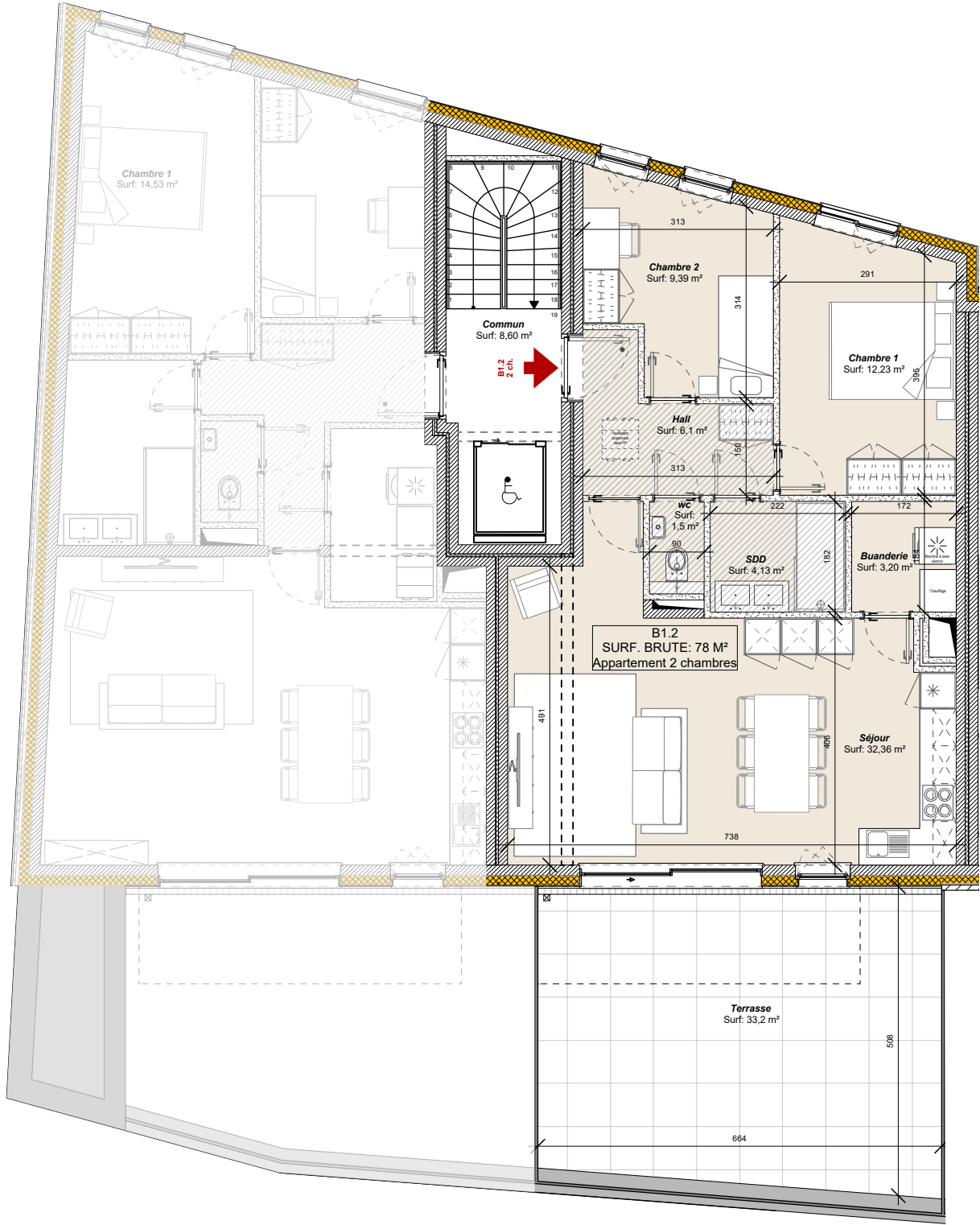
EXTRAIT DE PLAN DU 1er ETAGE APPARTEMENT B1.2
