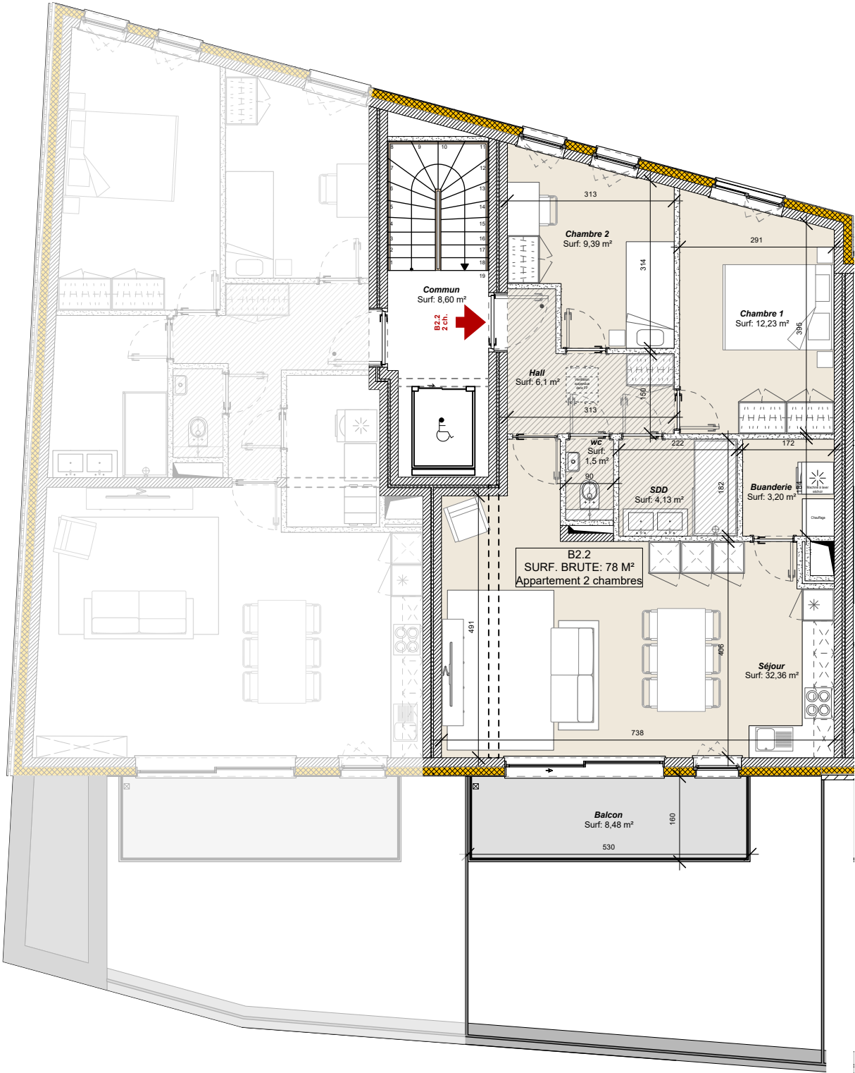
EXTRAIT DE PLAN DU 2e ETAGE APPARTEMENT B2.2
